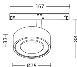
YAK207XX struttura bianco white structure
