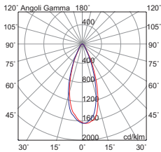
diagramma polare 7W 7W polar diagram
