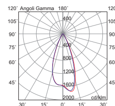
diagramma polare 13W 13W polar diagram
