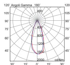
diagramma polare 7W 7W polar diagram
